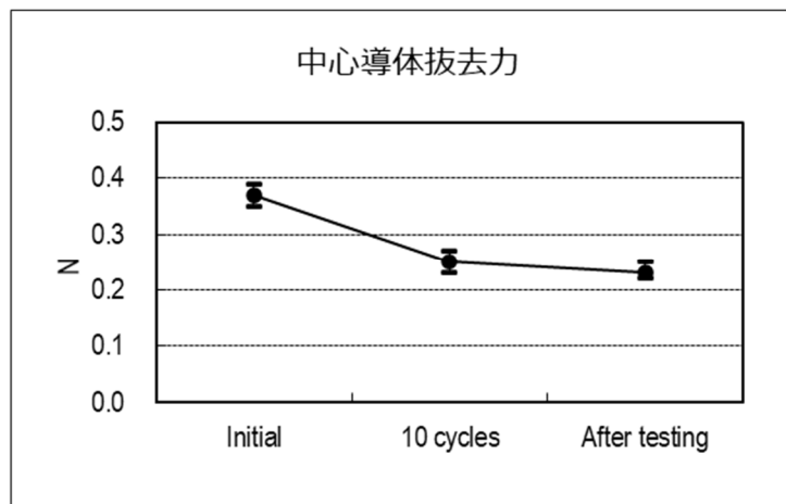
(グラフ 2) 抜去力
