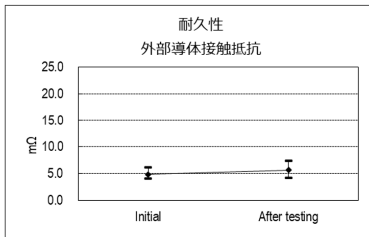
(グラフ 3) 耐久性
