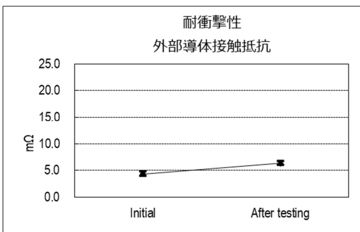
(グラフ 6) 耐衝撃性
