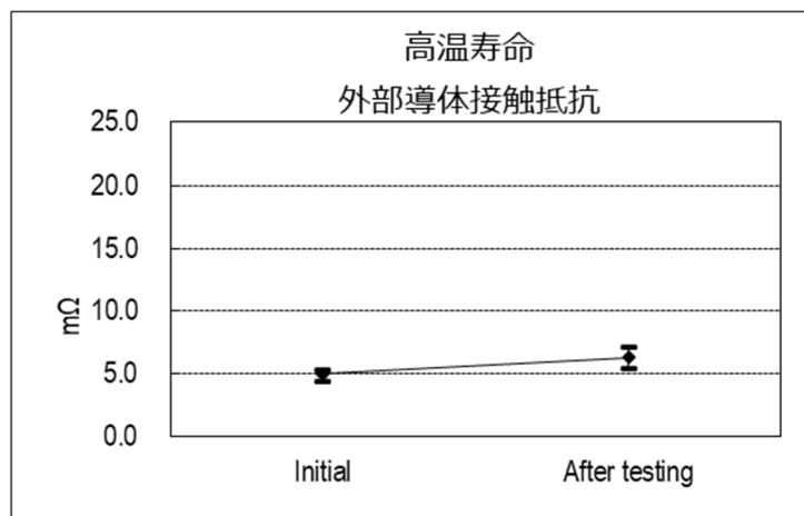
(グラフ 10) 高温寿命
