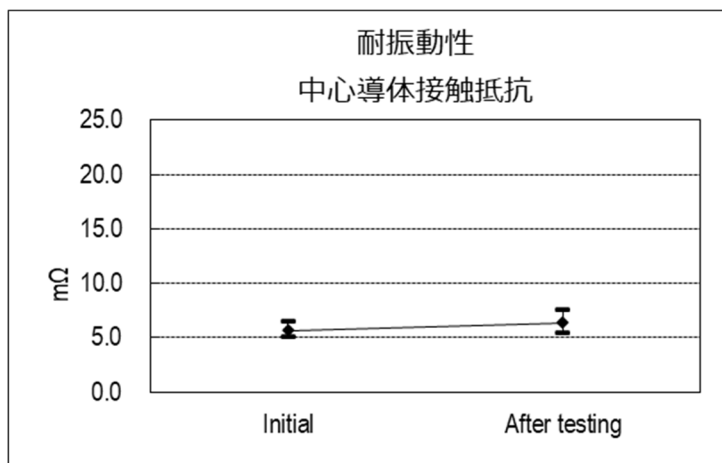
(グラフ 5) 耐振動性
