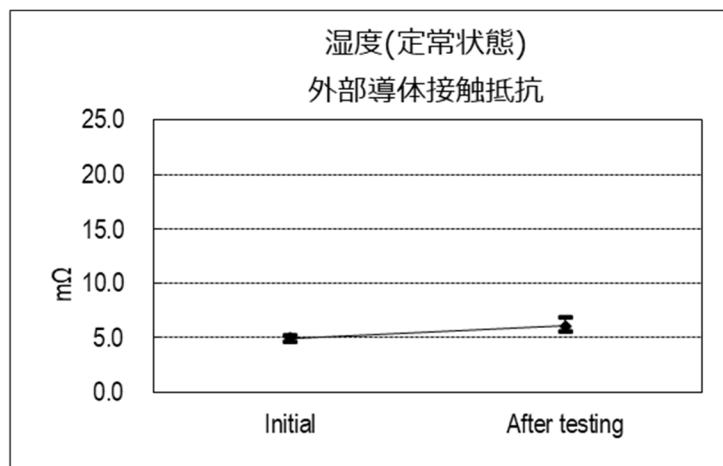
(グラフ 8) 湿度 (定常状態)
