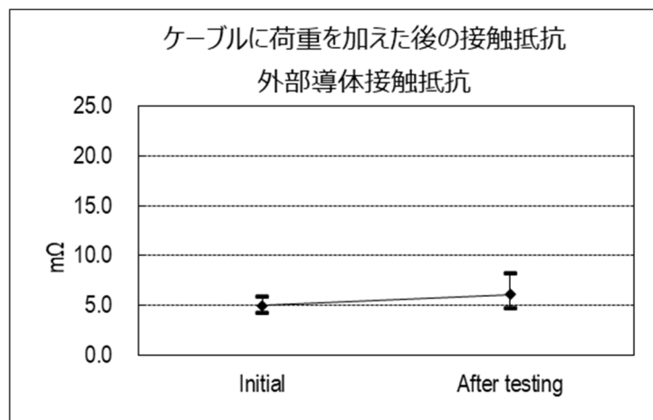
(グラフ 4) ケーブルに荷重を加えた後の接触抵抗
