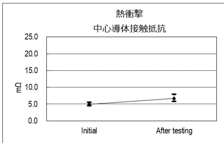
(グラフ 7) 熱衝撃
