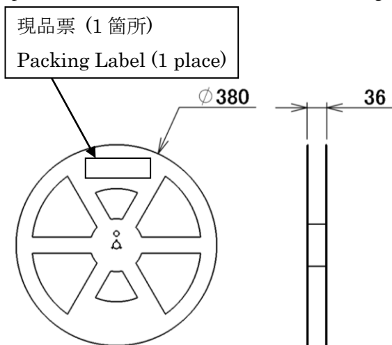
図 2.エンボスリール外径 Fig.2 Emboss reel diameter
