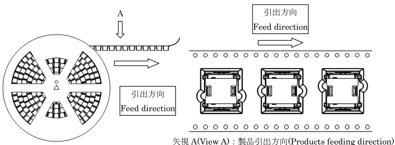
図 1.エンボスリール
