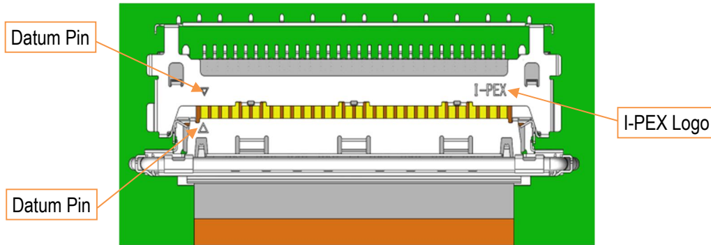
Fig. 4 Aligning Datum Pin Marks
