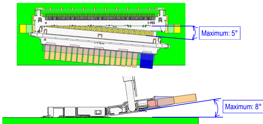
図.5 水平・垂直方向 最大挿入角度
