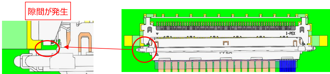
図. 6 半嵌合確認
