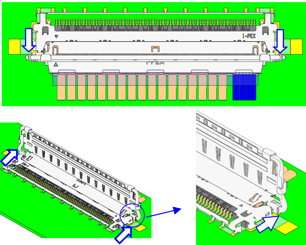
図. 21 抜去操作箇所
