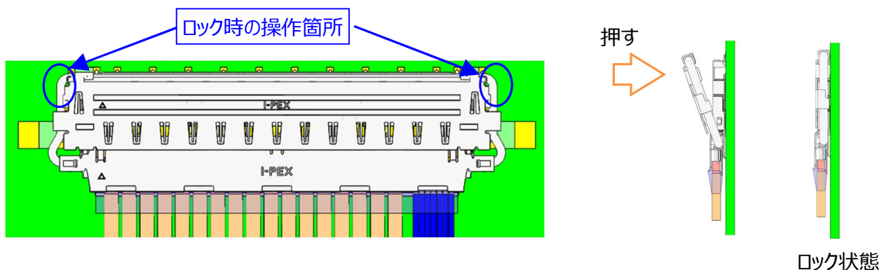
図. 16 嵌合ロック方法
