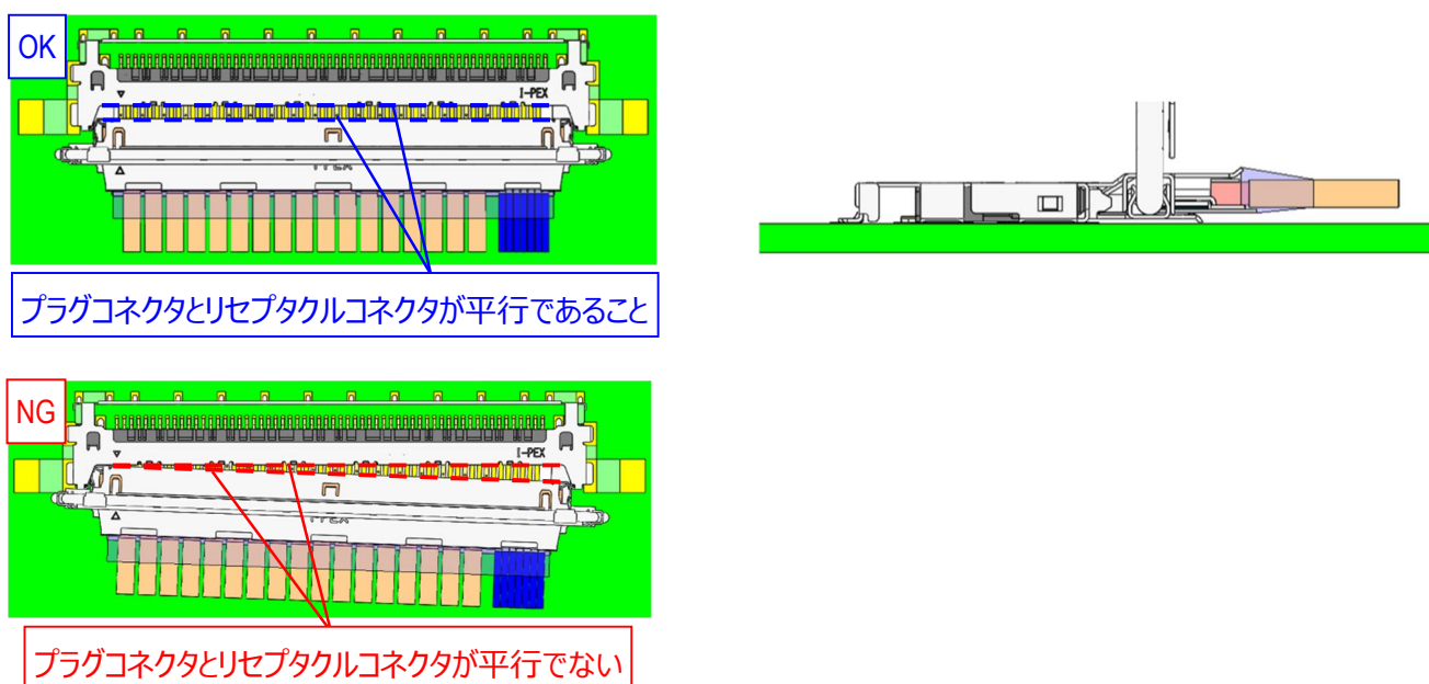
図.6 仮挿入完了状態
