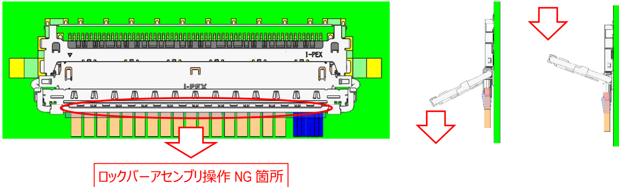
図. 23 抜去 NG 行為 1
