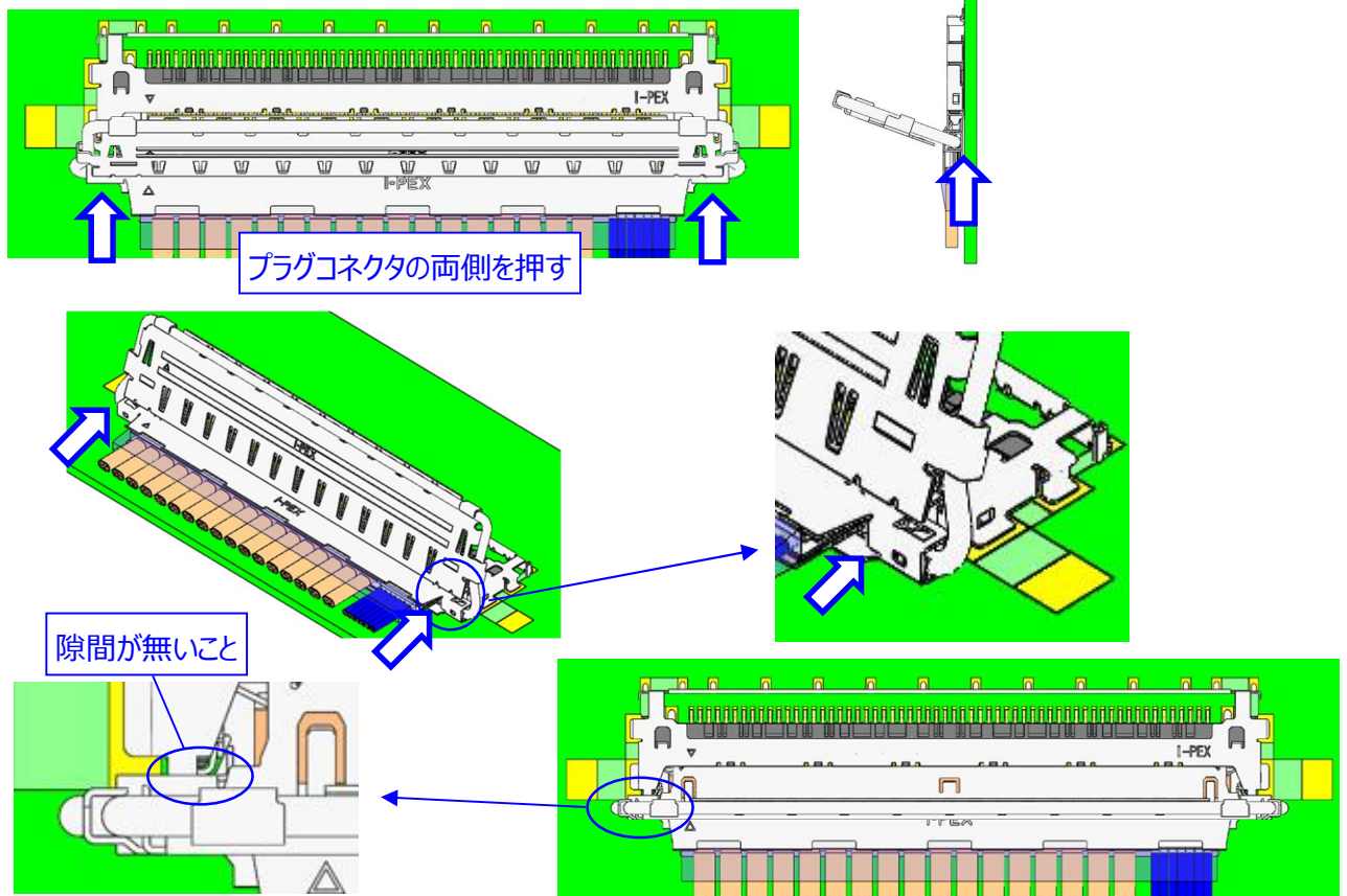
図. 5 プラグコネクタ挿入方法
