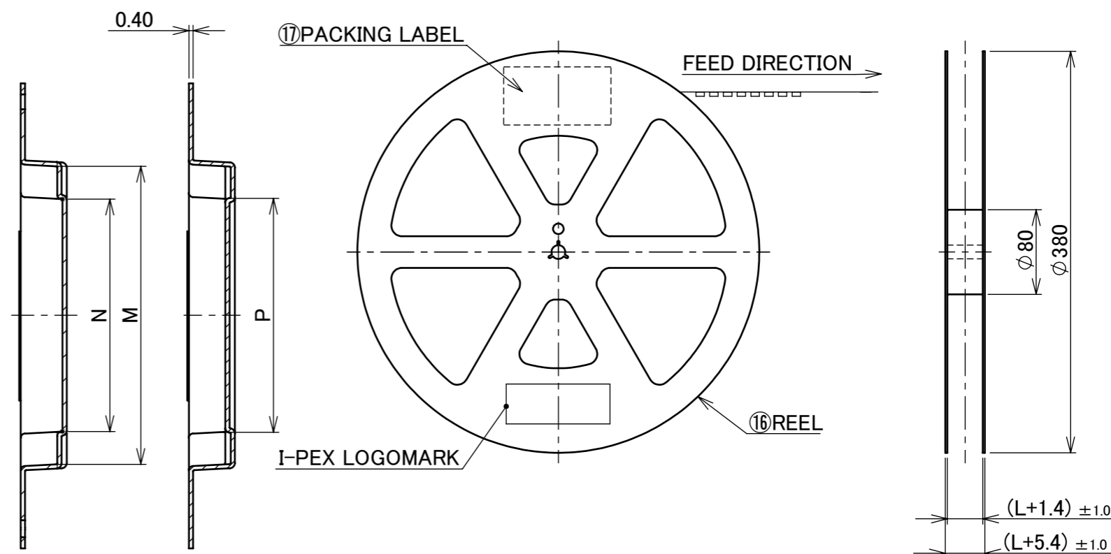
SECT. JJ-JJ (S = 2 : 1)
