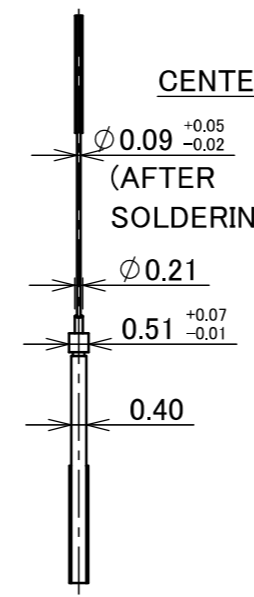
TWINAX CABLE AWG#40
