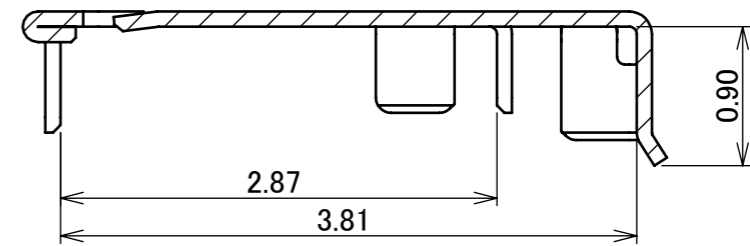
SECT.AA-AA (S=20/1)
